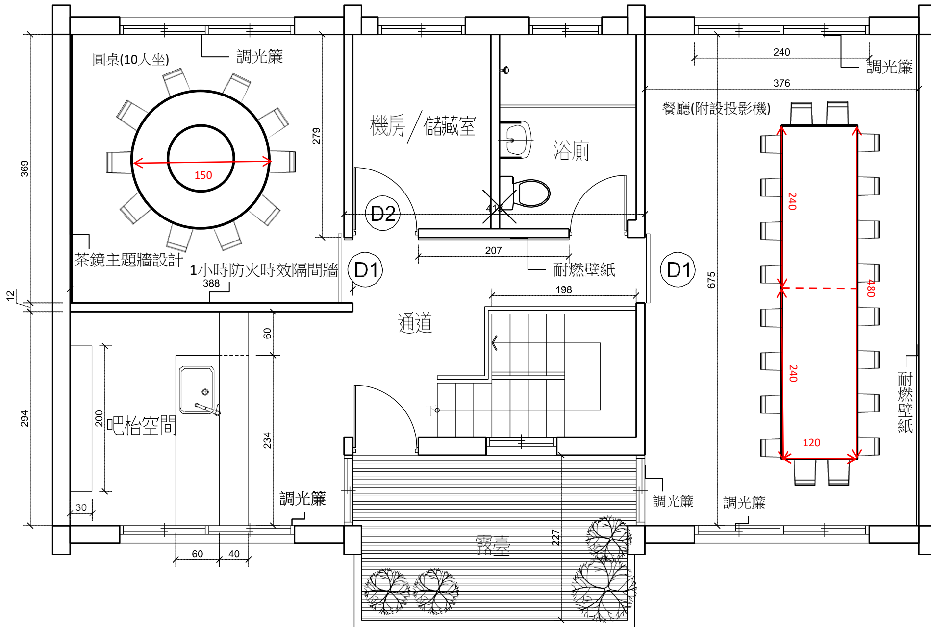
二樓(2902廳、2903廳、2904廳)
